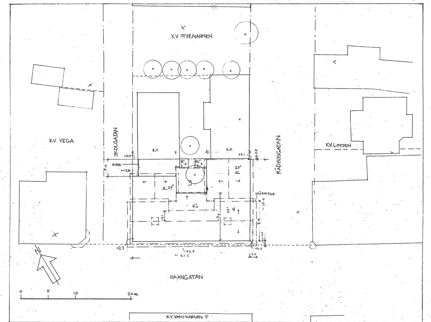
Situationsplan skala 1:400
