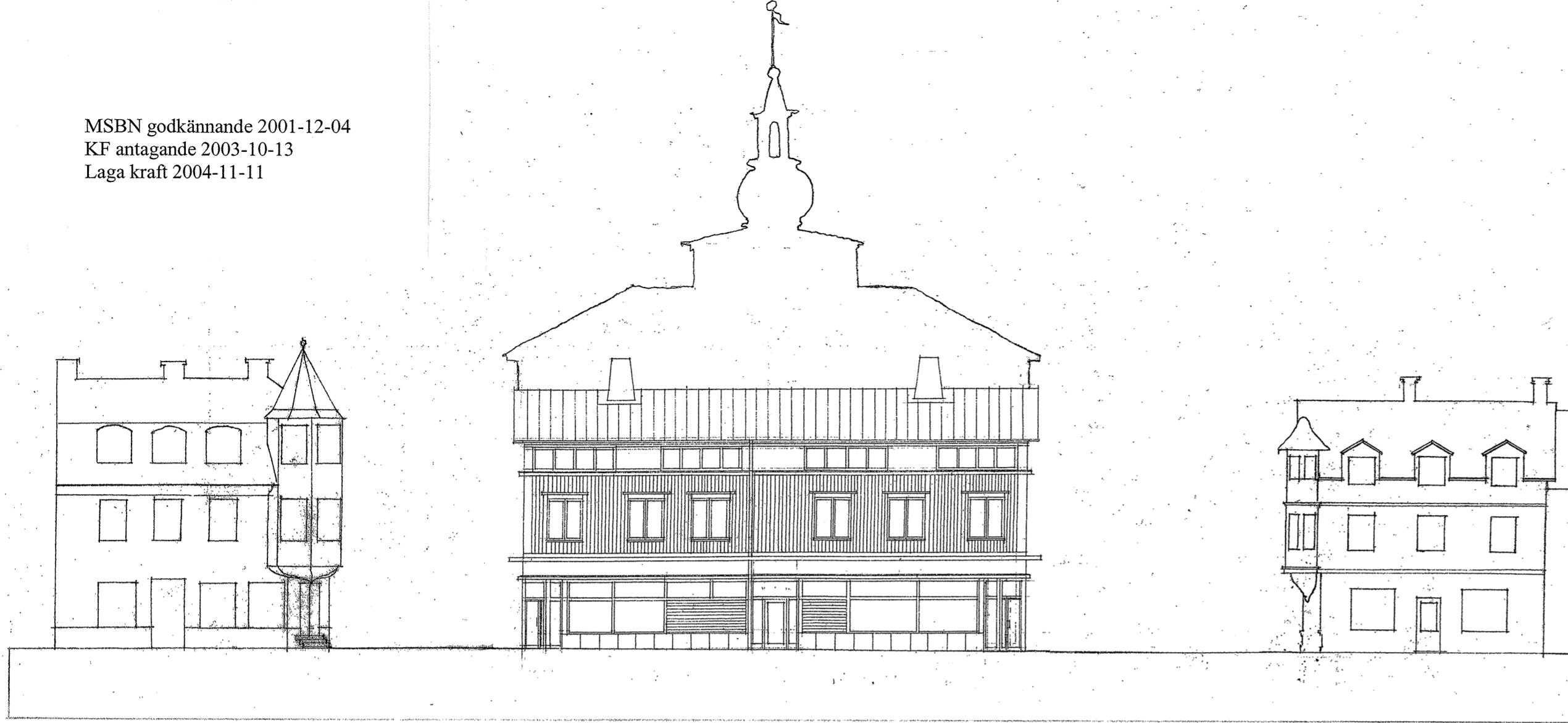
Fasad mot Hamngatan
