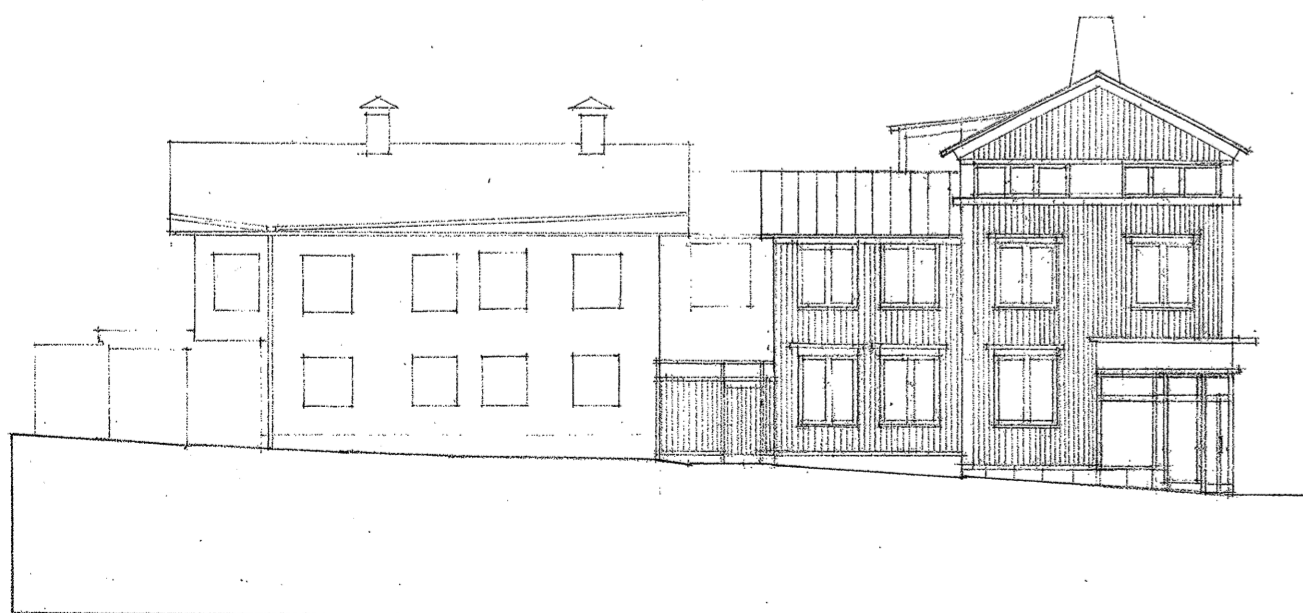
Fasad mot Skolgatan
